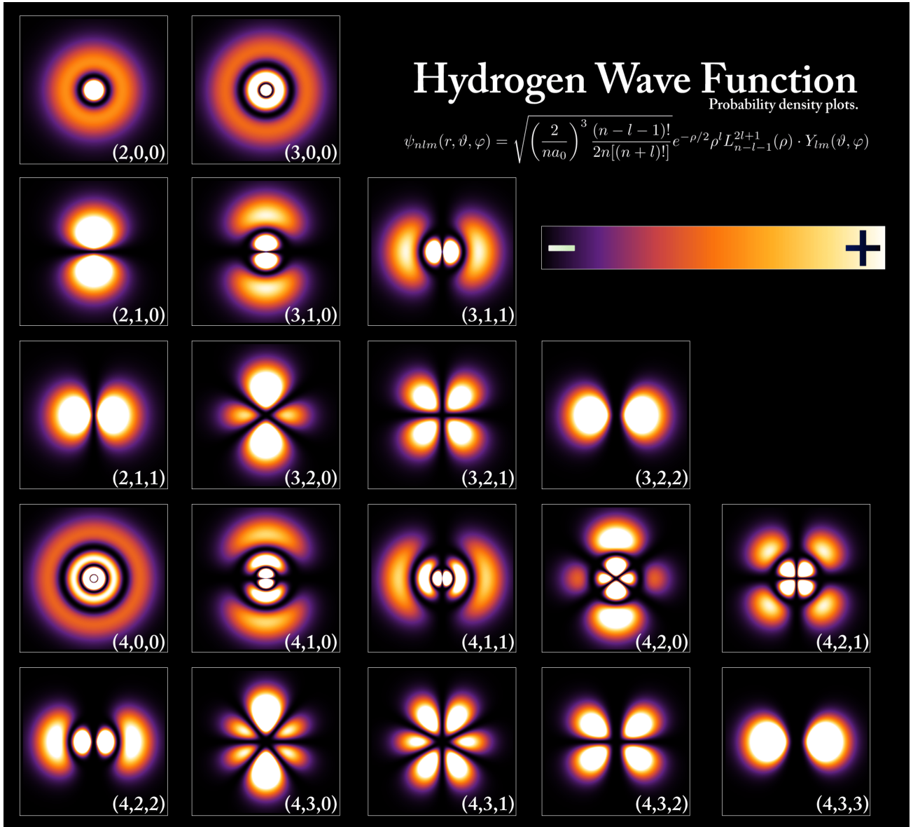
图 2 氢原子波函数
