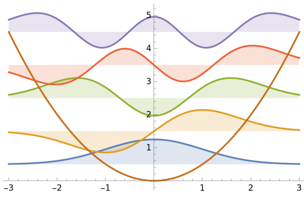
图 1 一维谐振子本征态
